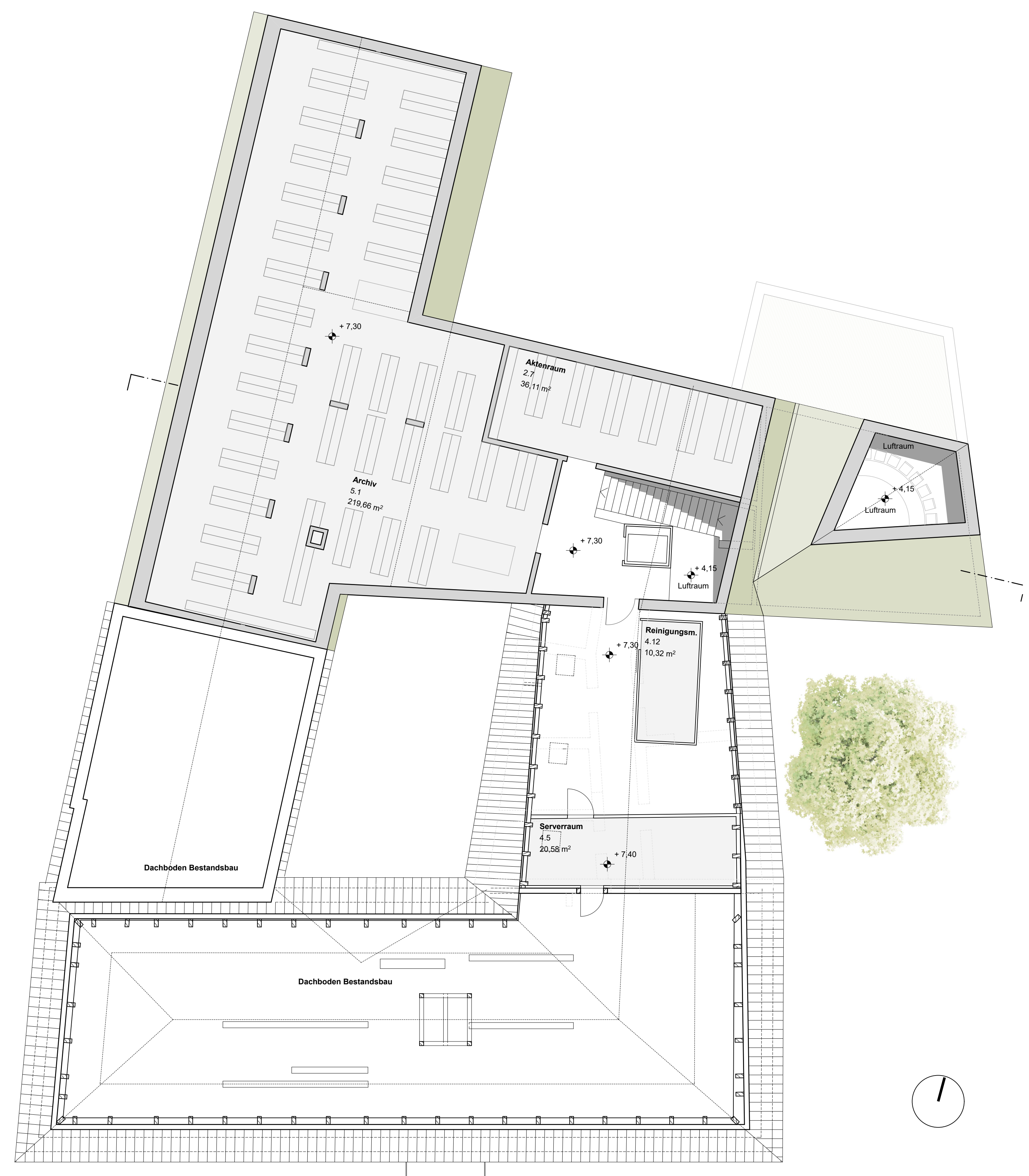
Grundriss DG, 1:100
