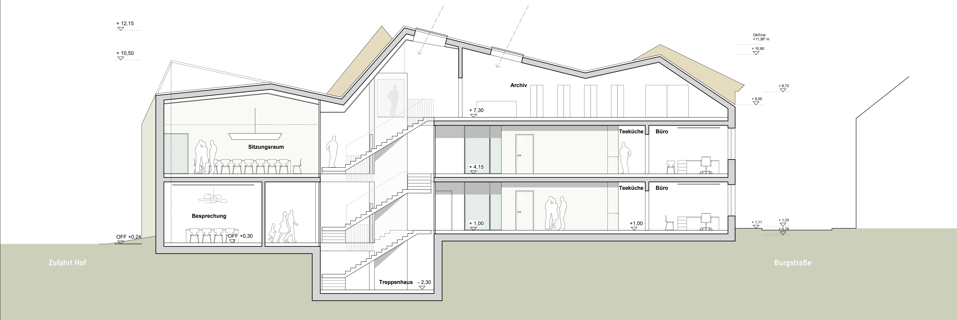
Schnitt, M 1:100
